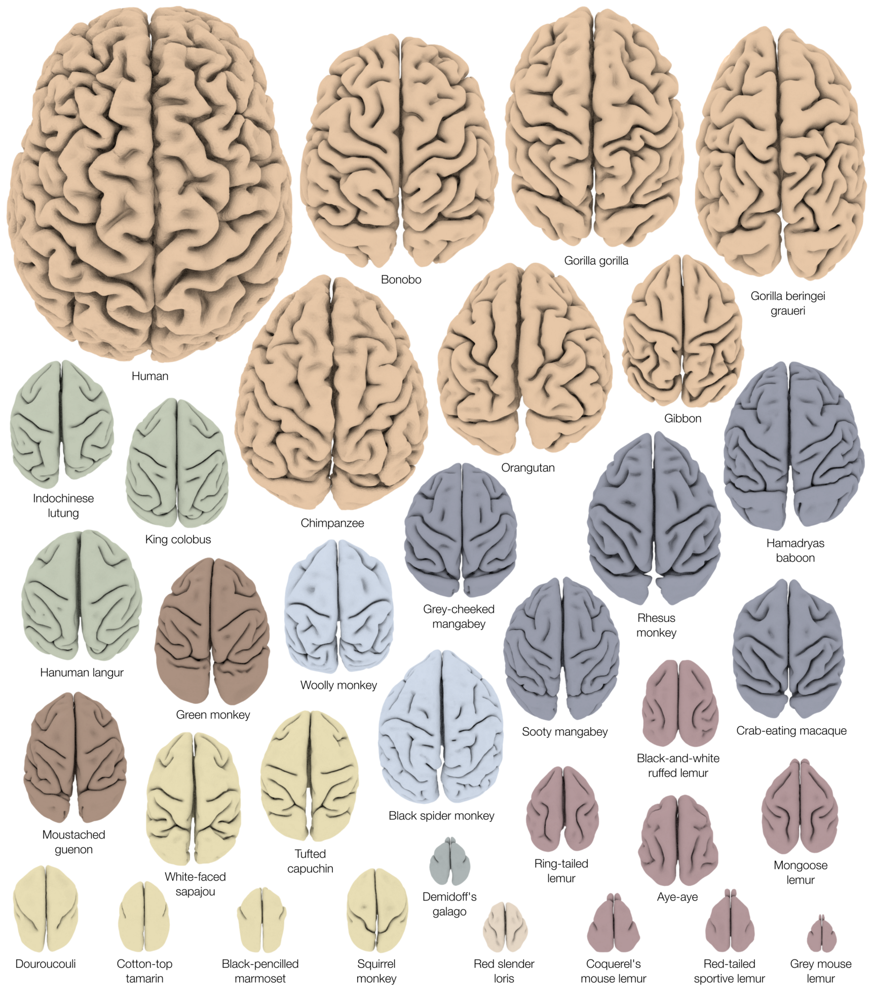
— Hominoidea — Colobinae — Papionini — Cercopitheciini — Atelidae — Cebidae — Galagonidae — Loridae — Lemuriformes 5 cm
