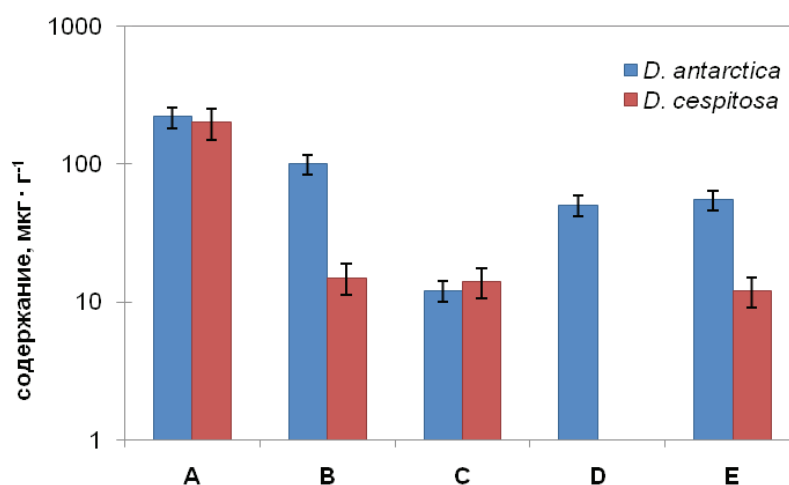
Рисунок. Содержание низкомолекулярных органических соединений в почве, в том числе: А – фенолов и фенолкарбоновых кислот, В – фенолкарбоновых кислот, С – гидроксibenзойных кислот, D – кумариновых производных и E – флавоноидов.
