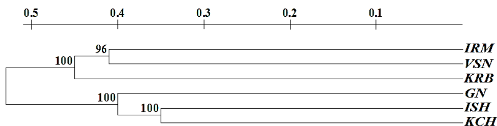
Рисунок 2. UPGMA-дендрограмма генетического сходства десяти изученных популяций L. sibirica , построенная на основании полиморфизма ISSR-маркеров. Шкала сверху — генетические расстояния; в узлах ветвления указаны значения бутстрепа (в %)
