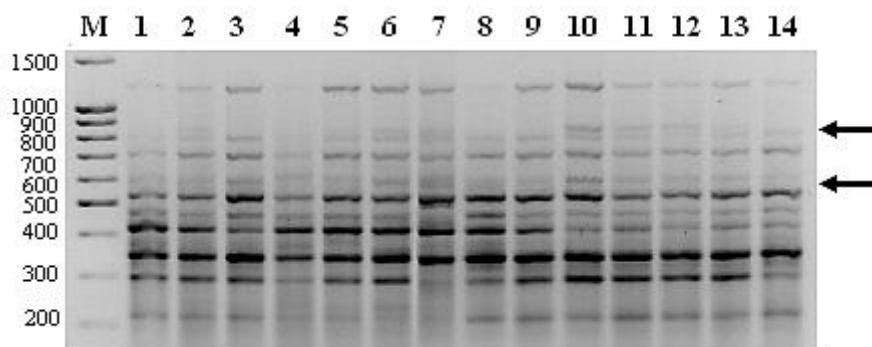
Рисунок 1. ISSR-спектр L. sibirica с праймером X10: М — маркер молекулярного веса, 1-14 — номера проб ДНК, стрелками обозначены некоторые полиморфные фрагменты.
