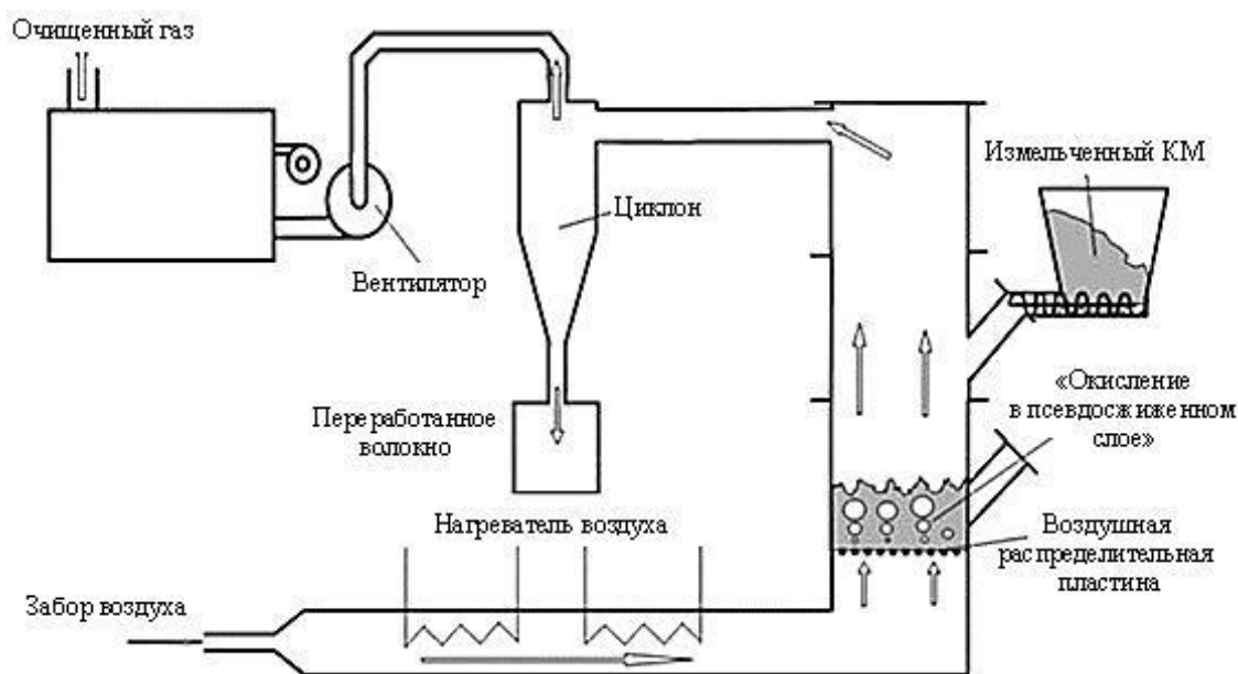
Рисунок 1. Принципиальная схема процесса сжигания ПКМ на основе углеродных волокон в высокотемпературном псевдооживленном слое [2]
