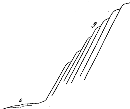
Skematisk profil, visande sandstensens (s) läge i förhållande till protogingneisen (g) vid Husqvarna.
