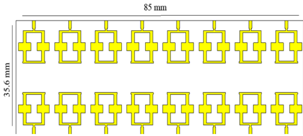
Fig. 6 Dimension of 8x2 linear array antenna
