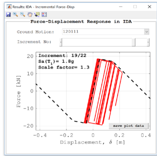
(d) Force-Displacement at SA increments
