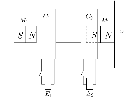
Fig. 33: Generator
