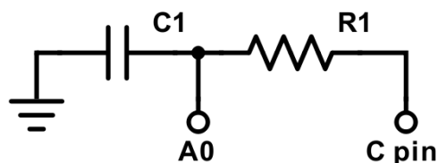
Slika 1, Sa C pin je označen pin preko koga se puni kondenzator (eng. charge pin ), C1 je nepoznata kapacitivnost, A0 analogni ulaz, R1 je otpornik u RC kolu (ovde 10 kΩ).
