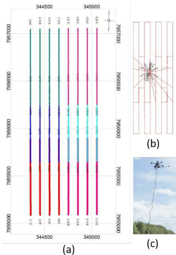
FIGURA 7 - Planejamento de voo para aquisição de dados magnetométricos por drone: a) Disposição das linhas de aquisição de dados; b) plano de voo adquirido com ponto de lançamento; c) detalhe do equipamento geofísico magnetômetro, adaptado ao drone, para aquisição de dados.
