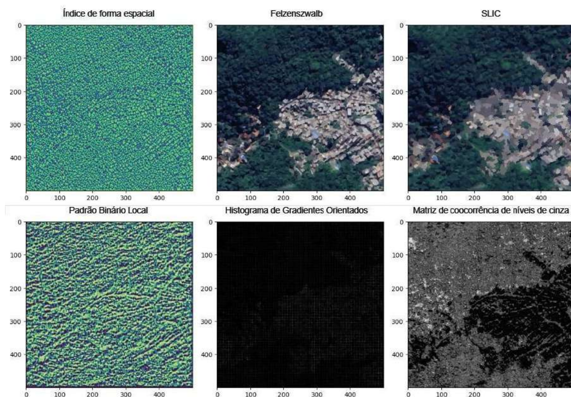
FIGURA 2 - Da esquerda para a direita, de cima para baixo: índice de forma espacial; média dos superpixels de Felzenszwalb; média dos superpixels SLIC; LBP; representação visual do HOG; representação visual da GLCM. Elaboração própria.
