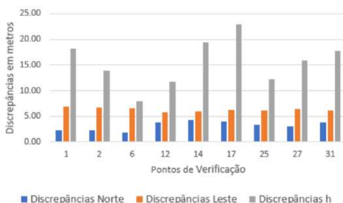
FIGURA 6 – Gráfico das discrepâncias dos pontos de verificação em C5. Fonte: Rodrigues (2023).
