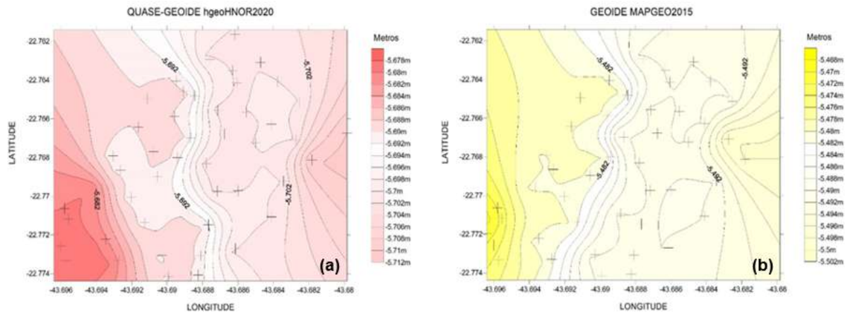
FIGURA 6 – Modelos: (a) do quase-geóide (hgeoHNOR2020) e (b) do geóide (MAPGEO2015). Elaboração própria.
