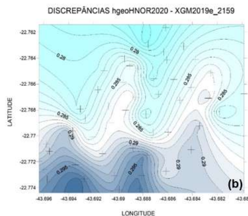
FIGURA 10 - Modelo de discrepâncias entre (a) o hgeoHNOR2020 e MGG EGM2008 e (b) o hgeoHNOR2020 e o MGG XGM2019e_2159. Elaboração própria.
