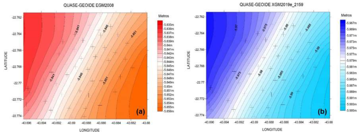
FIGURA 7 - Modelos do quase-geóide (a) do EGM2008 e (b) do XGM2019e_2159. Elaboração própria.
