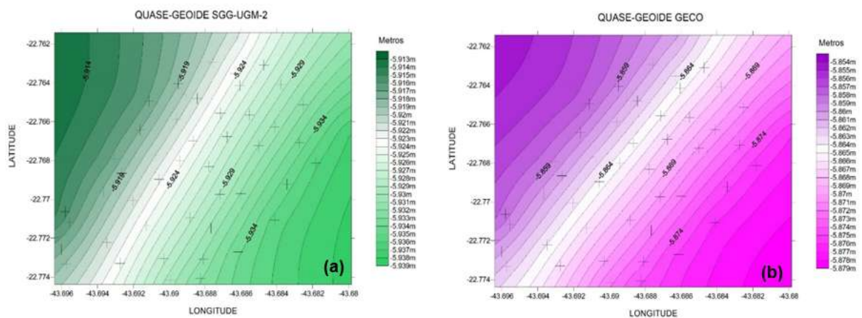
FIGURA 8 - Modelos do quase-geóide (a) do SGG-UGM-2 e (b) do GECO. Elaboração própria.
