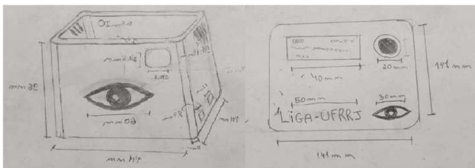
FIGURA 3 - Diagrama esquemático atualizado, feito à mão, da caixa do módulo de sensoriamento, a ser modelada computacionalmente e impressa em impressora 3D. Fonte: Maria Santos.
