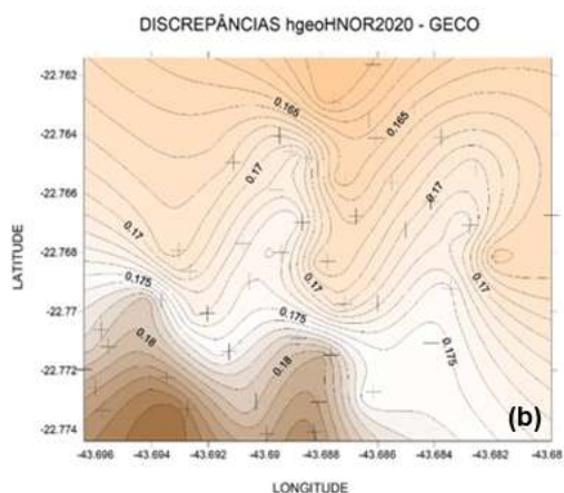
FIGURA 11 - Modelo de discrepâncias entre (a) o hgeoHNOR2020 e o MGG SGG-UGM-2 e (b) o hgeoHNOR2020 e o MGG GECO. Elaboração própria.
