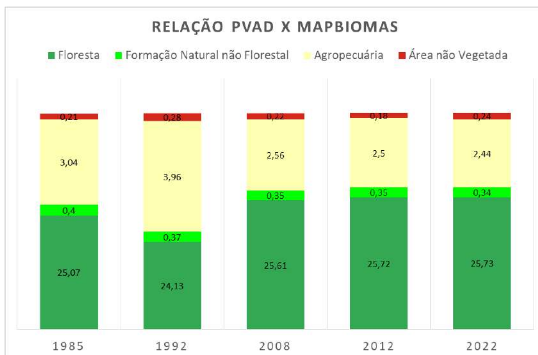
FIGURA 4 - Gráfico mostrando a área (km 2 ) ocupada por cada relação entre o Argissolo Vermelho-Amarelo Distráfico (PVAd) e MapBiomas. Fonte: IBGE e MapBiomas.
