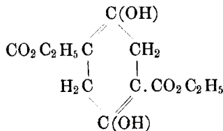
Δ 1,4 Dioxydihydroterephthalsäureäther.
