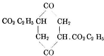
Diketohexahydroterephthalsäureäther
