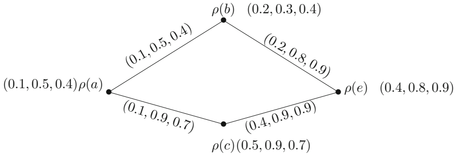
Fig. 26 Food web
