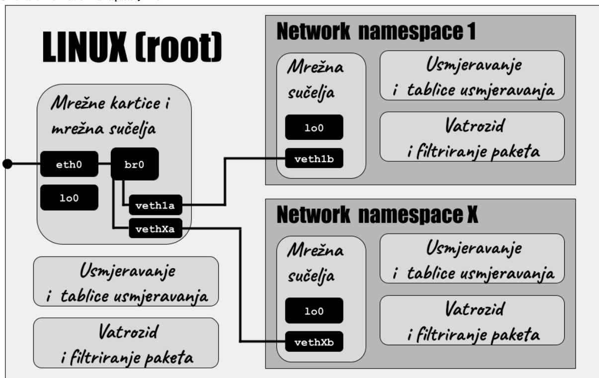
Slika 40.A. Linux network namespaces → Linux
