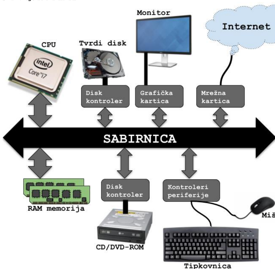
Slika 41. Logička shema računala.
