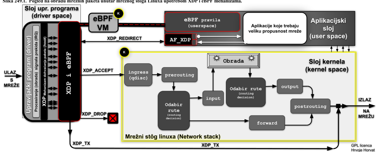
Slika 249.1. Pogled na obradu mrežnih paketa unutar mrežnog stoga Linux a upotrebom XDP i eBPF mehanizama.
