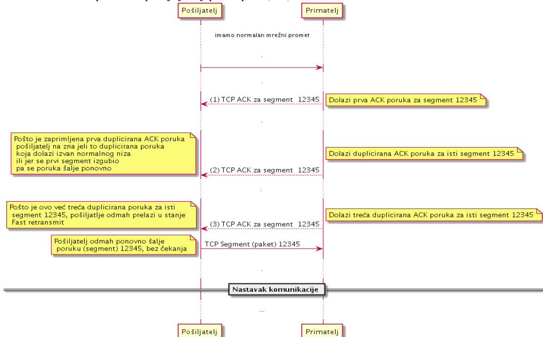
Slika 219. Prikaz rada TCP protokola kod ponavljanja slanja potvrđne poruke ( ACK ).
