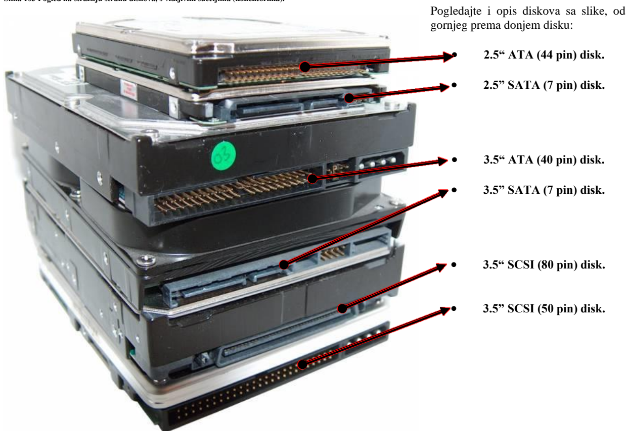
Slika 103 Pogled na stražnju stranu diskova, s vidljivim sučeljima (konektorima).
