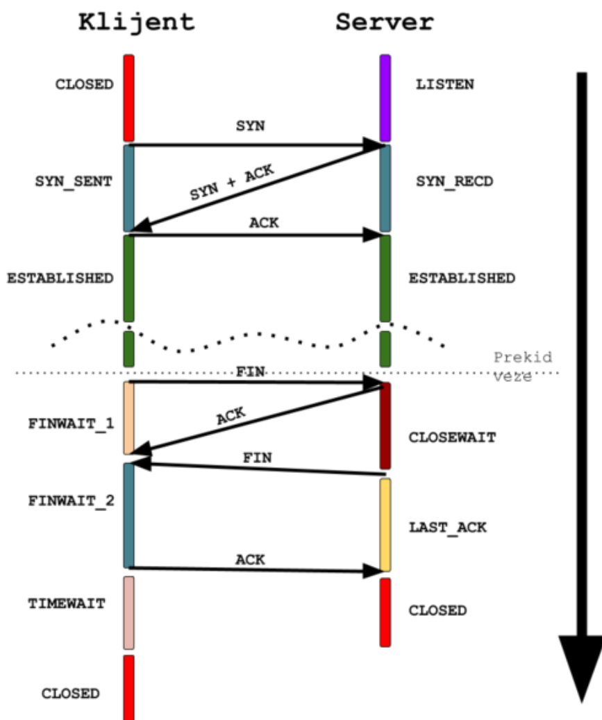
Slika 227. Stanja TCP veze klijenta i poslužitelja.
