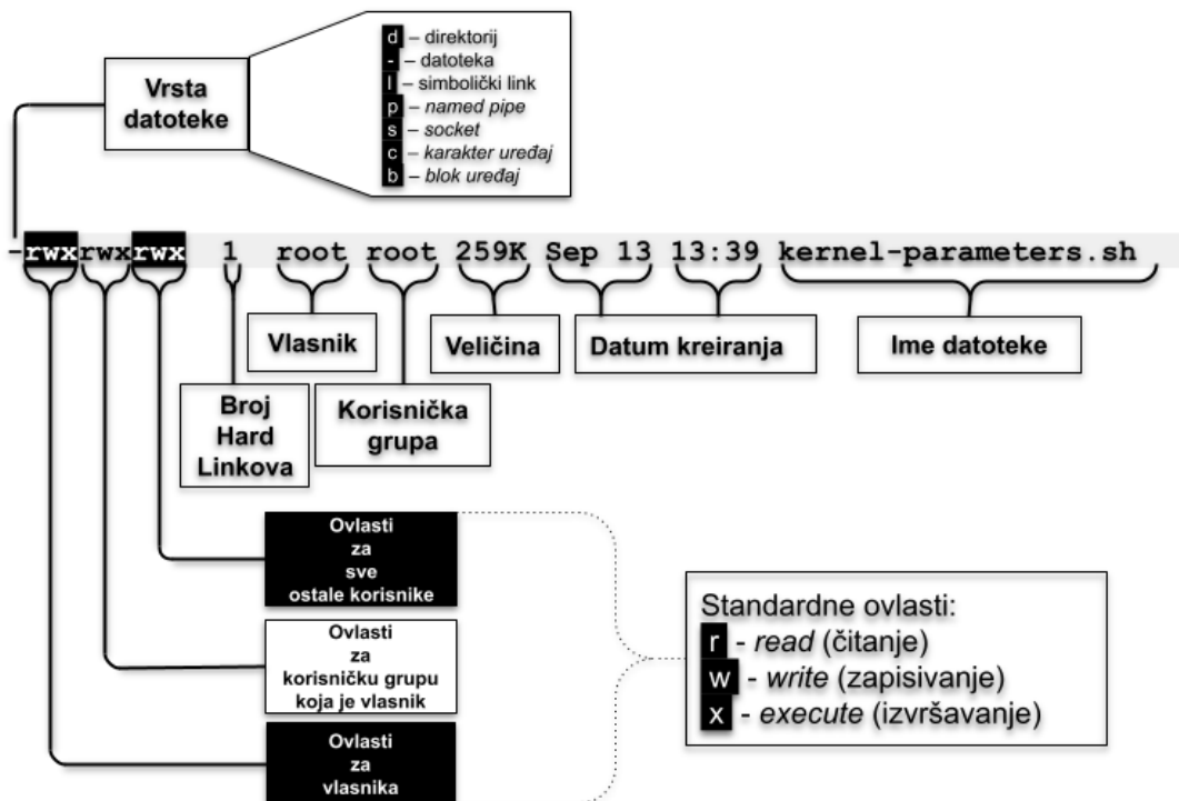
Slika 8.1. Sažeti pogled na ovlasti.
