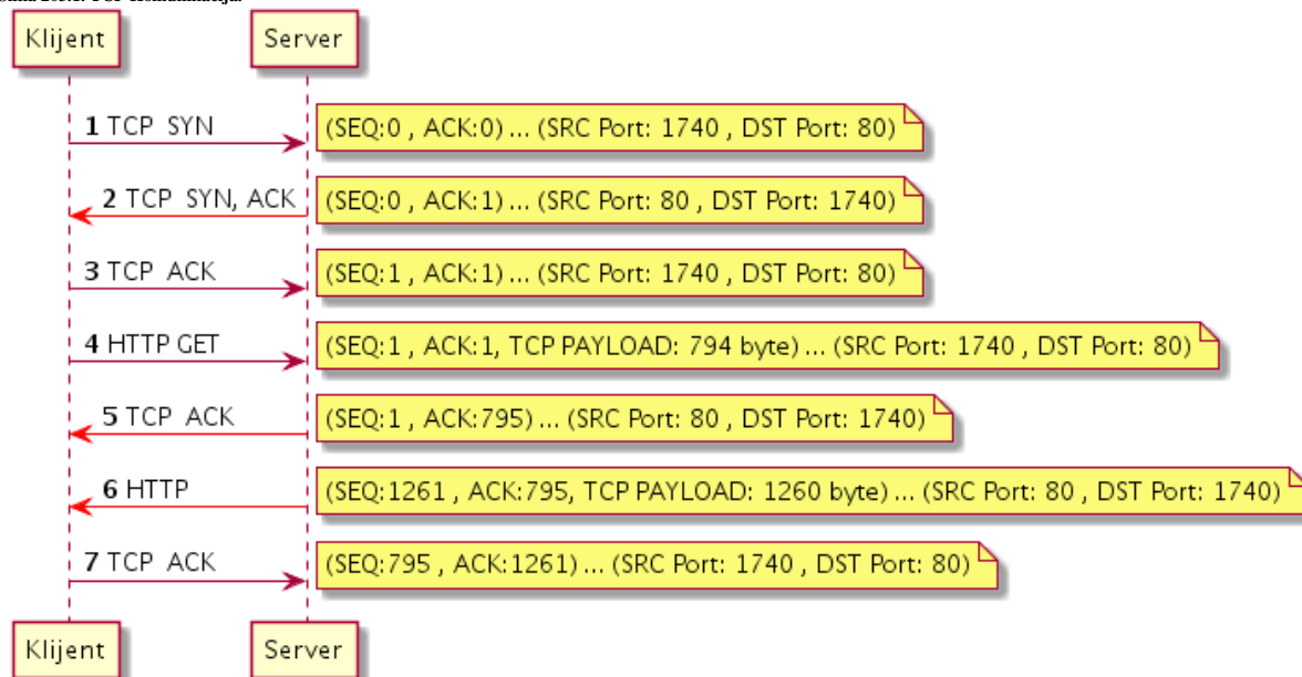
Slika 203.1. TCP Komunikacija.
