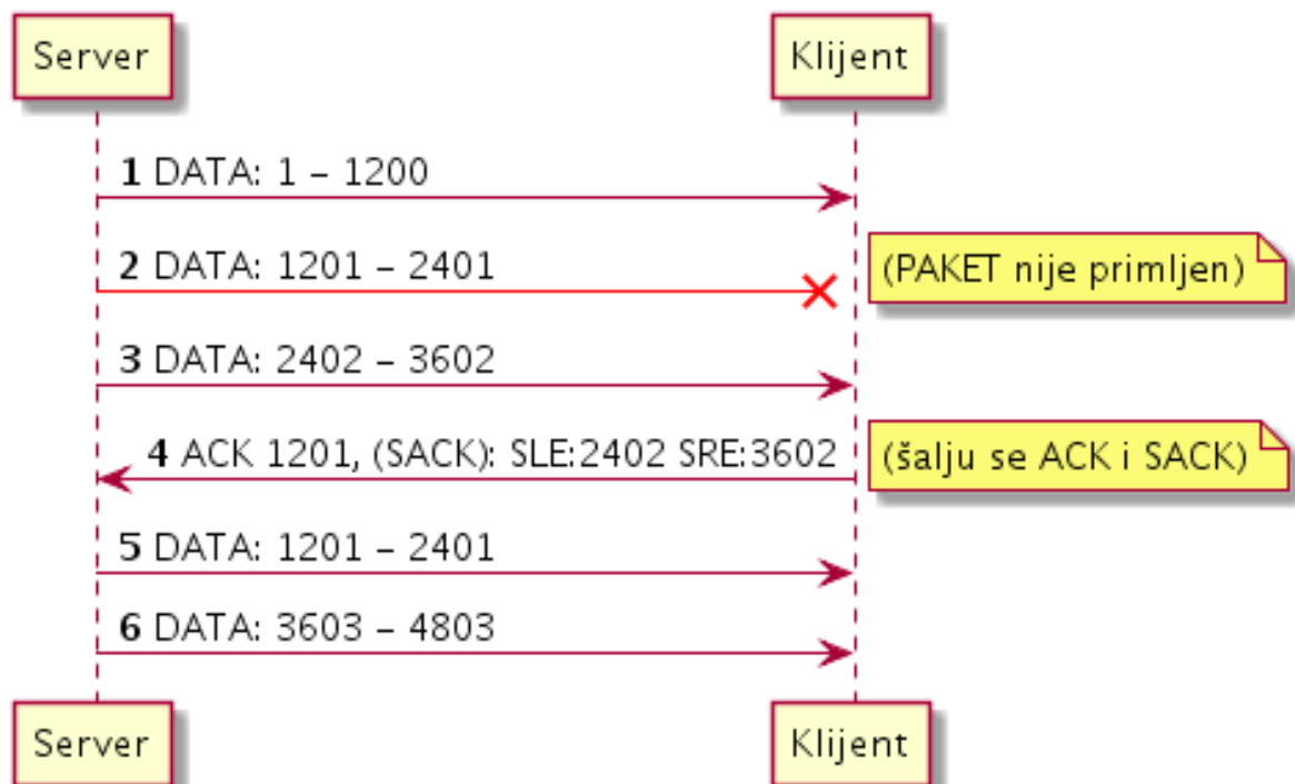
Slika 204. TCP komunikacija sa SACK porukama.
