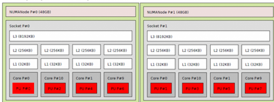
Slika 70. Logički izgled Intel Xeon E5606 procesora
