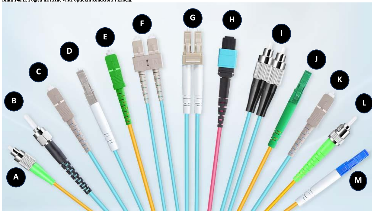
Slika 148.L. Pogled na razne vrste optičkih konektora i kabela.
