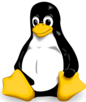
Slika 79. Pingvin TUX
