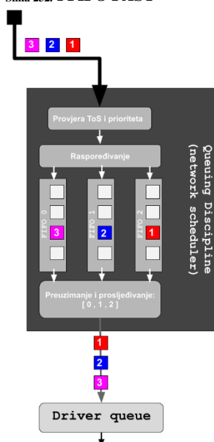
Slika 232. PFIFO FAST
