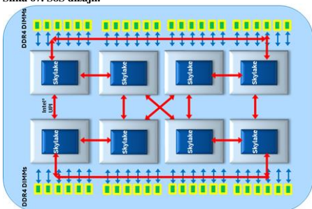
Slika 67. S8S dizajn.
