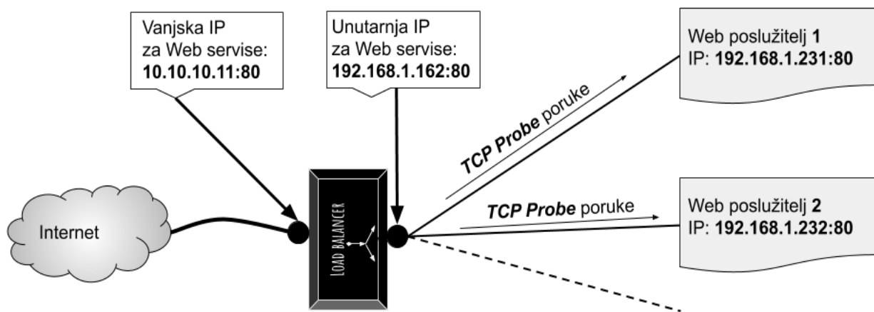
Slika 224.2. TCP Probe poruke koje šalje Load Balancer prema web poslužiteljima kako bi periodički provjeravao jesu li dostupni (živi).
