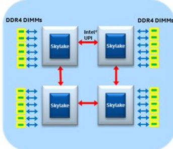
Slika 65. dolje: S4S (prstenasti spoj:2xUPI)
