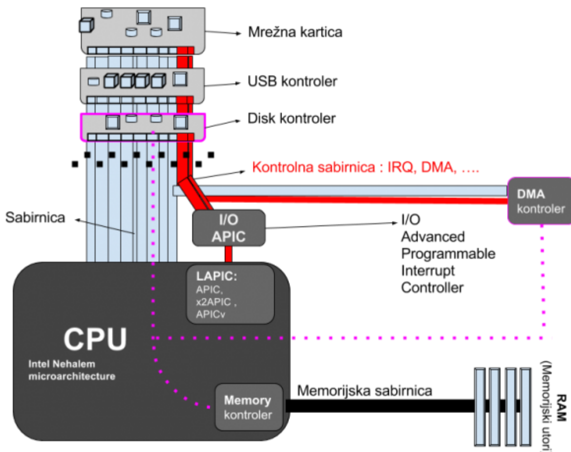
Slika 54. Logička arhitekturnalna shemu IRQ i DMA podsustava: komunikacija
