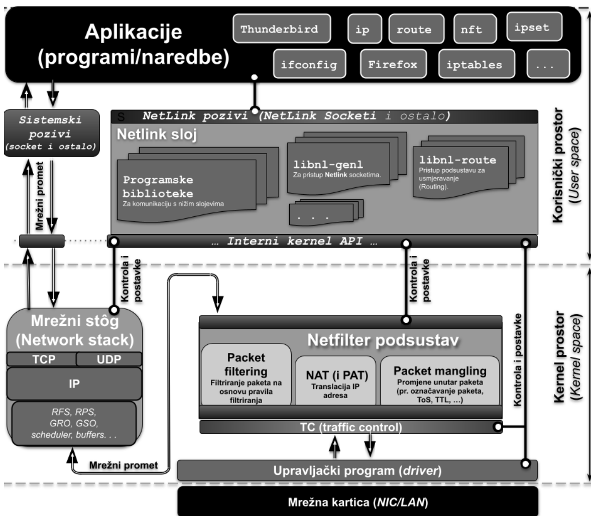
Slika 228. Mrežni model Linuxa.
