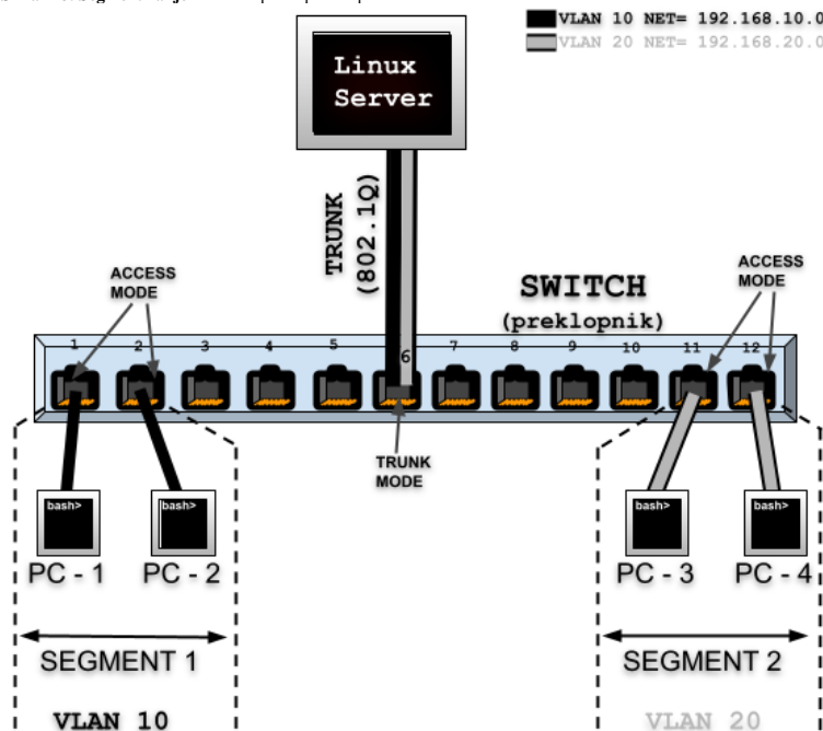
Slika 173. Segmentiranje mreže na preklopniku upotrebom VLAN ova.
