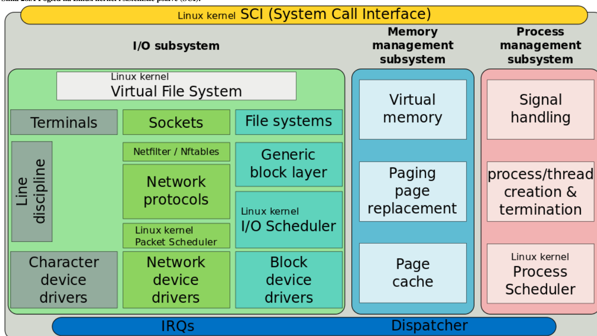
Slika 28.A Pogled na Linux kernel i sistemске pozive (SCI):
