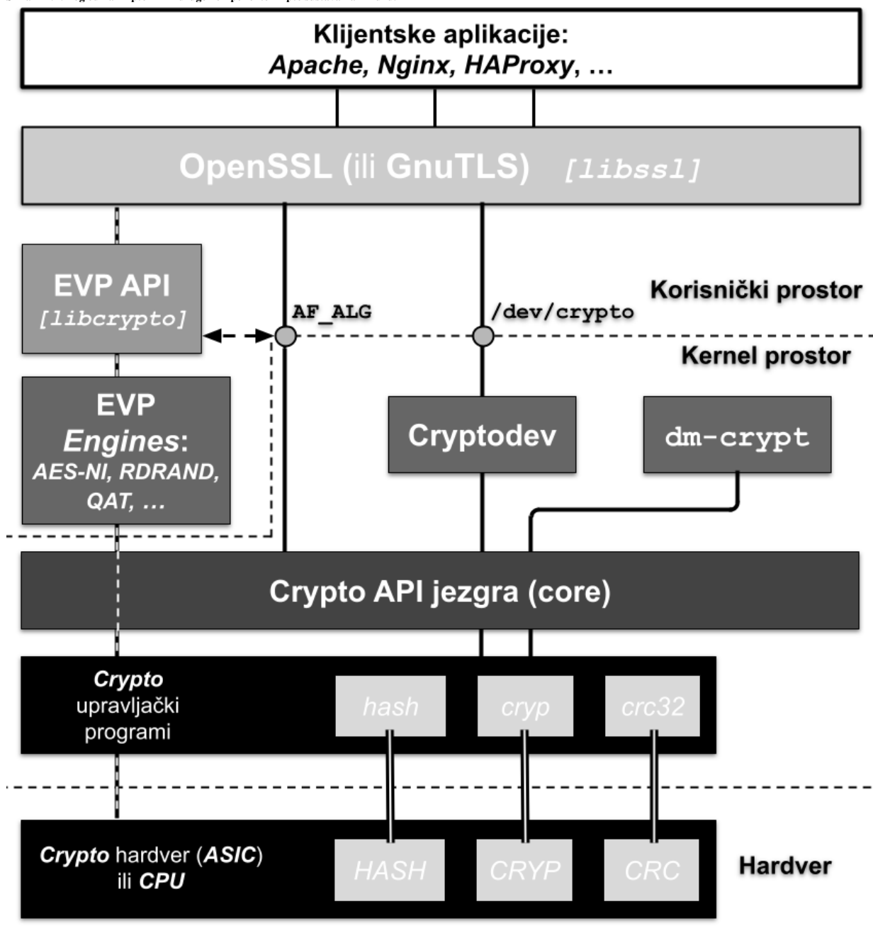
Slika 244.F. Pogled na kriptografski API i druge komponente kriptografskog sustava na Linuxu.
