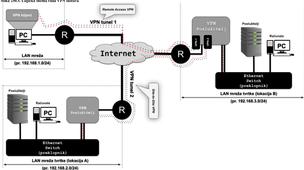
Slika 250.5. Logička shema rada VPN sustava
