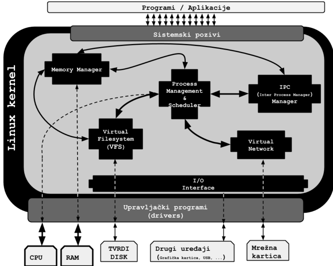
Slika 80. Pogled na logičku shemu Linux kernela.
