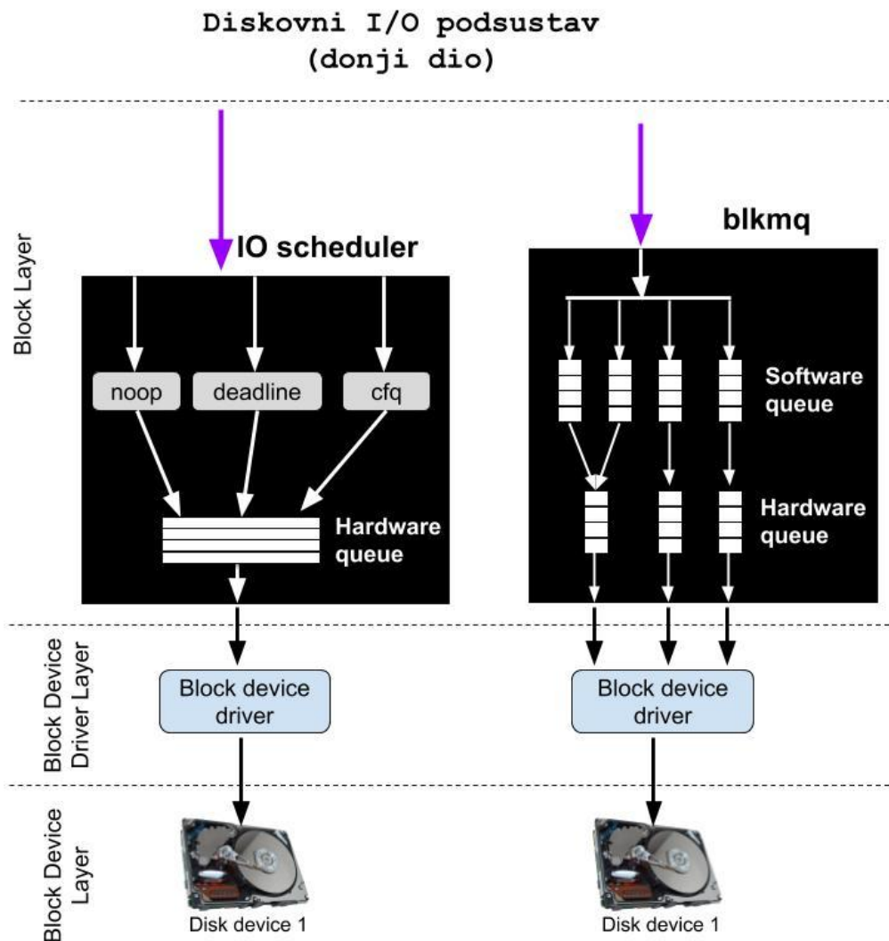
Slika 133. Pogled na blkmq komponentu.
