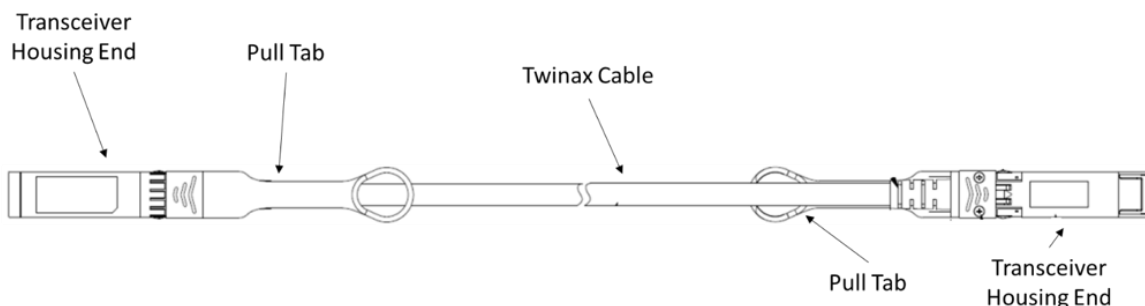
Slika 145.4. SFP DAC s Twinax kabelom
