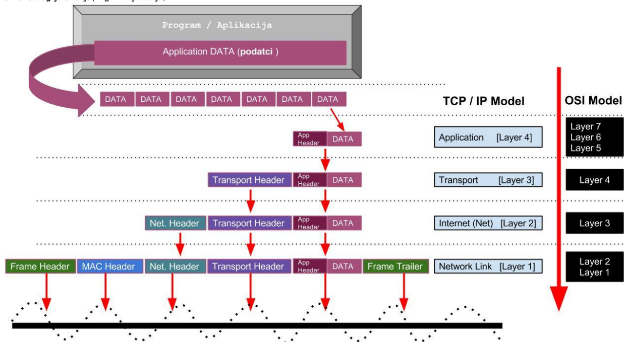
Slika 159. Ugnježdvanje (Engl. Enkapsulacija )
