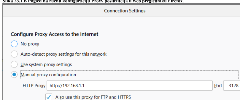
Slika 23.1.B Pogled na ručnu konfiguraciju Proxy poslužitelja u web pregledniku Firefox.
