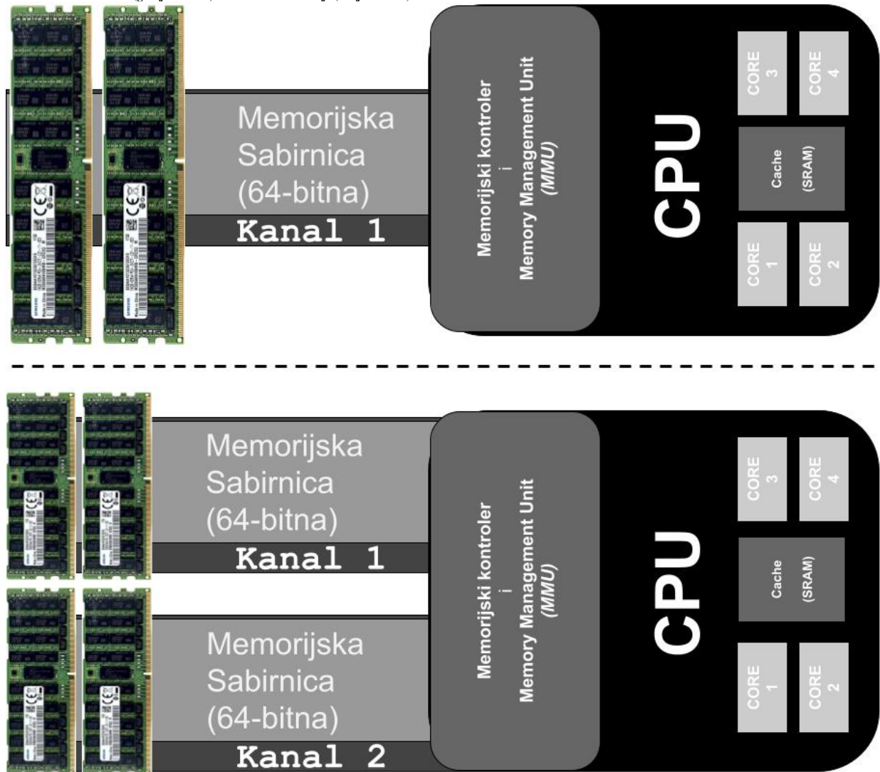
Slika 92.C. Jednokanalna (gornji dio slike) i Dvokanalna memorija (donji dio slike)
