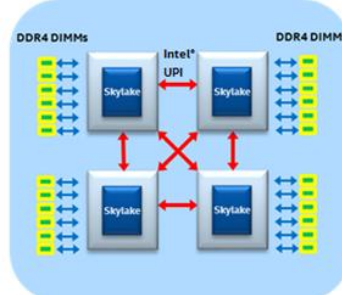
Slika 66. dolje: S4S (unakrsni spoj: 3xUPI)
