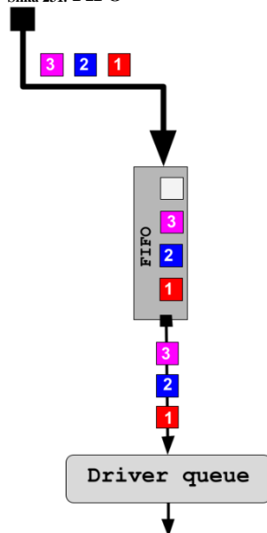
Slika 231. FIFO
