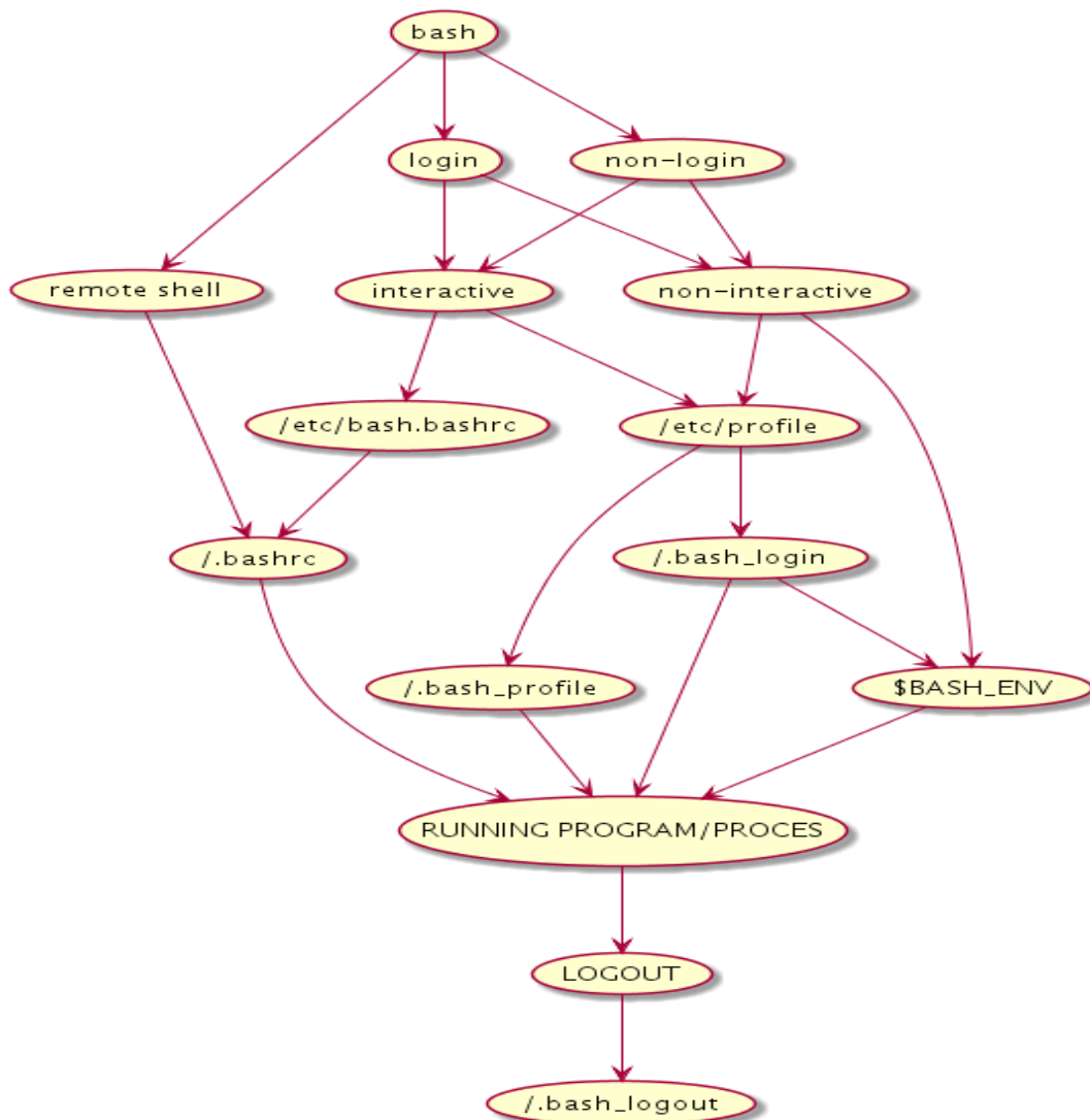
Slika 6. Bash ljuska.
