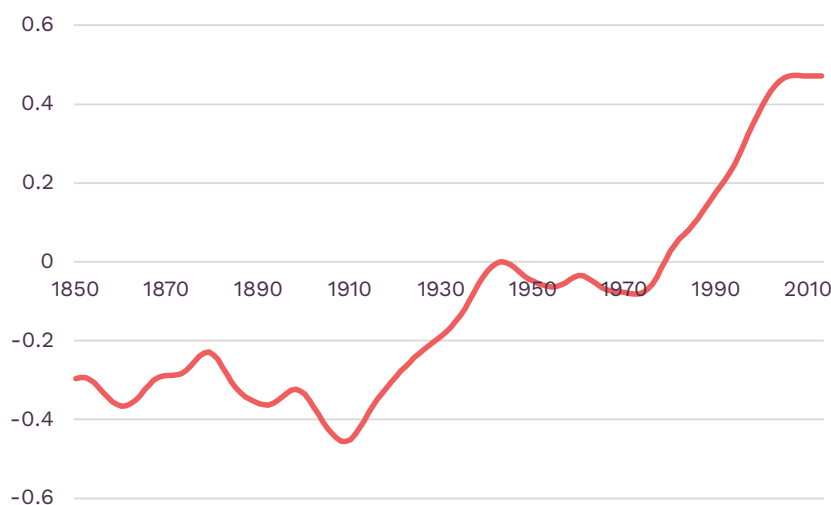
Figure 2.16 Global temperature, 1850-2010 (°C)
