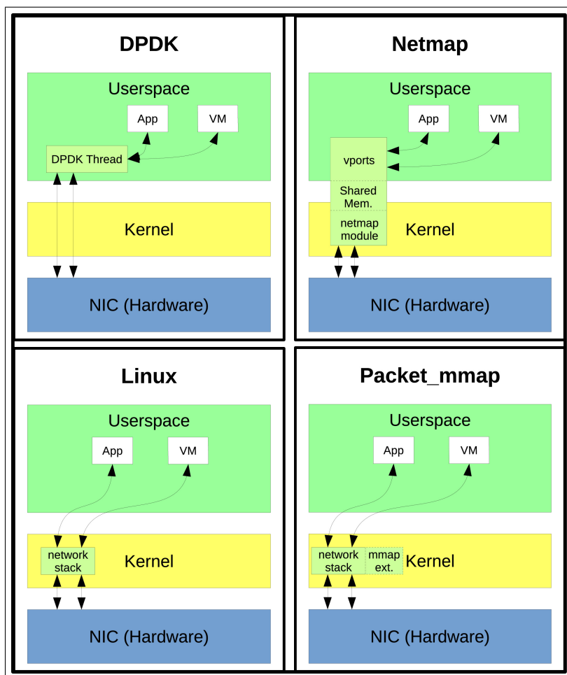
Figura 1. Comparação entre a arquitetura dos sistemas testados
