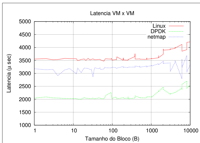
Figura 4. Teste de latência entre duas VMs
