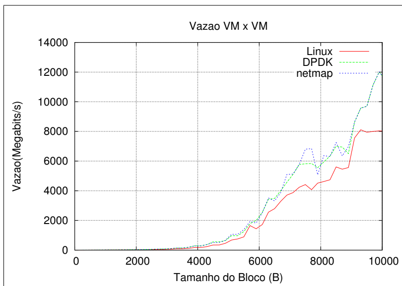
Figura 3. Teste de vazão entre duas VMs
