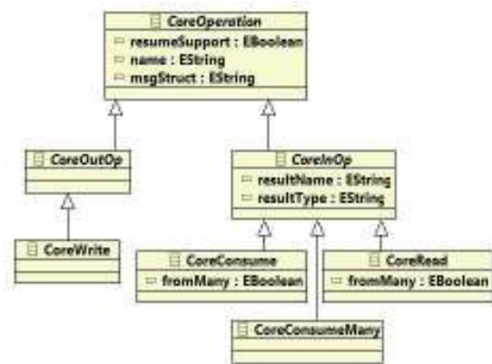
Fig. 5. The corecl meta-model
