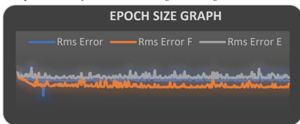
Fig. 4 Epoch size
