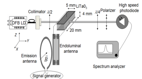
Fig.1 : Schéma d'expérience de capteur de champ magnétique par cristal Electro optique
