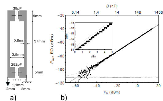
Fig.2 : a) capteur de base b) Courbe de Linéarité
