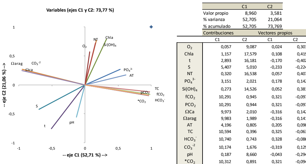
Figura 6. Representación gráfica del análisis de componentes principales aplicados a los parámetros del sistema carbónico en aguas del Golfo de Cariaco.
