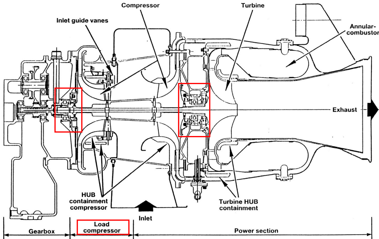
APU GTCP36-300
