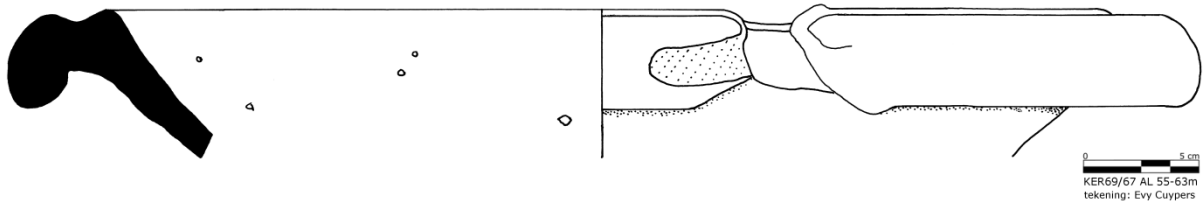
Profieltekening van het mortarium randfragment RAMS00383
