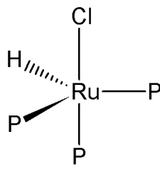
axial-(Cl),cis
