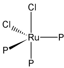
axial,cis
