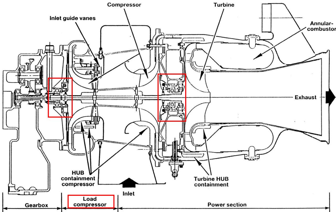
APU GTCP36-300
