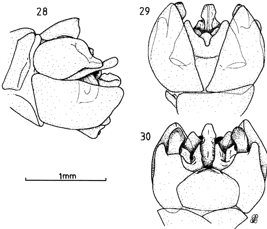
Figs 28–30. Diocobroma flavotermatum Hull, holotype male genitalia. 28. Lateral. 29. Ventral. 30. Dorsal.
