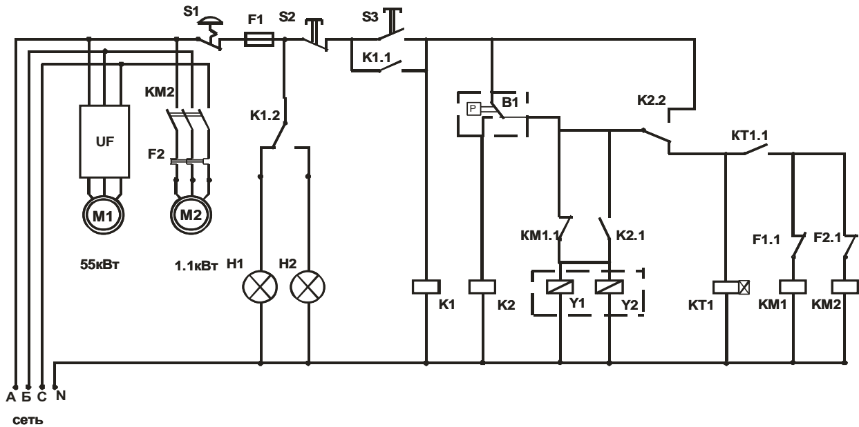
Рисунок 1. Электрическая схема пуска компрессорного агрегата по предлагаемой системе: UF-устройство плавного пуска или частотный преобразователь; M1-двигатель компрессора; M2- двигатель вентилятора; H1, H2-кантрольные лампы; K1, K2-промежуточные реле управления; Y1, Y2-клапана продувки и всасывания; KT1-реле времени; KM1, KM2-электромагнитные пускатели.
