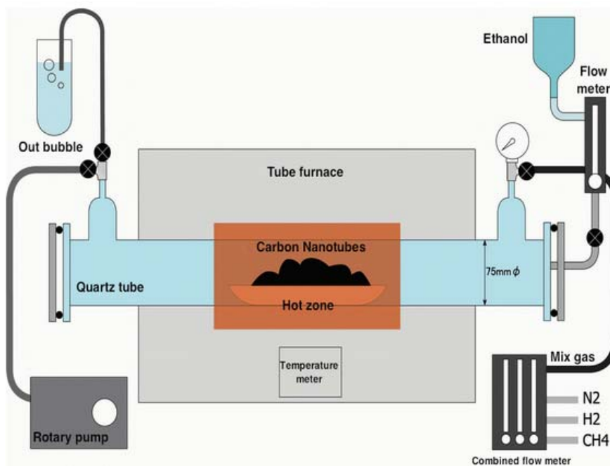
Fig. 6 CVD [13]
