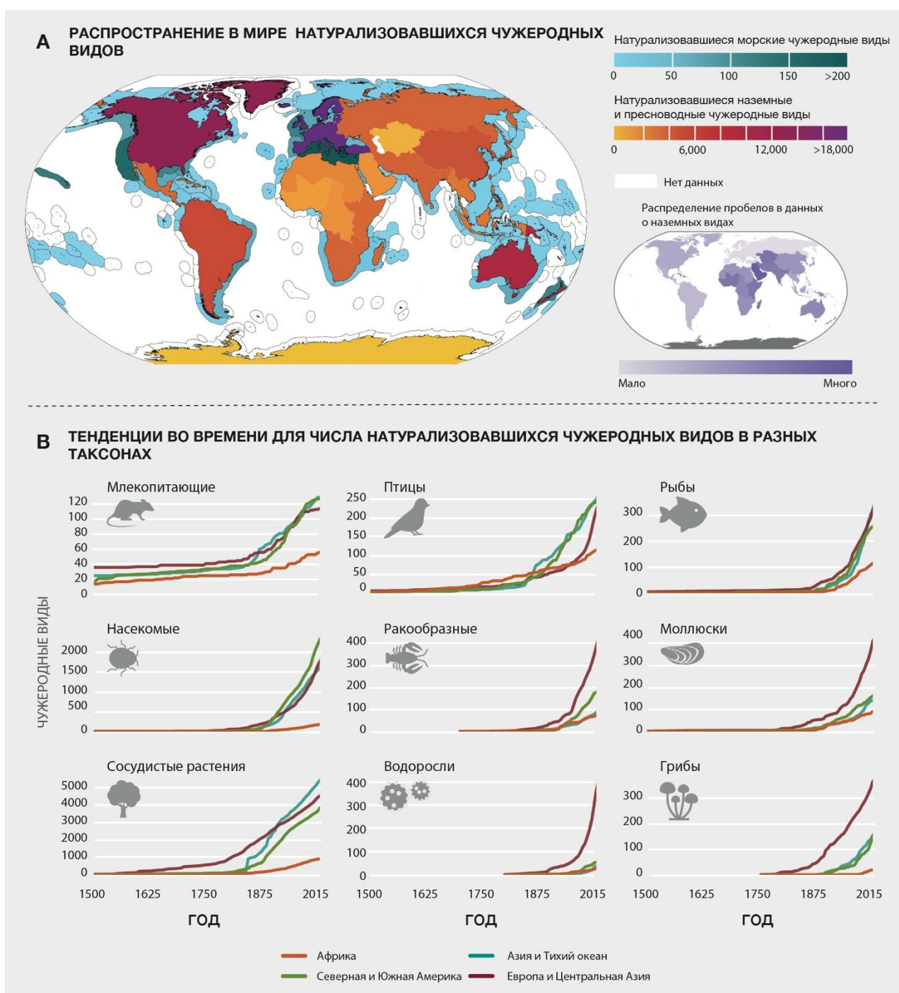
Рис. РДО.4. Распространение в мире и тенденции во времени у натурализовавшихся чужеродных видов. (А) Указано общее число натурализовавшихся чужеродных видов (наземные и пресноводные виды) в 18 субрегионах МПБЭУ и в морских экологических регионах (морские виды). Белым цветом обозначено отсутствие информации {2.2}. Для выявления пробелов в данных был проведен анализ пробелов для наземных регионов, как показано на вставке {2.1.4, 2.2.3}. Анализ пробелов в данных не удалось провести для морских регионов (белый цвет) и Антарктики (серый цвет). (В) Тенденции изменения числа натурализовавшихся чужеродных видов во времени (с 1500 по 2015 год) показаны для млекопитающих, птиц, рыб, насекомых, ракообразных, моллюсков, сосудистых растений, водорослей и грибов в четырех регионах МПБЭУ {2.1.4, 2.4.1}.
