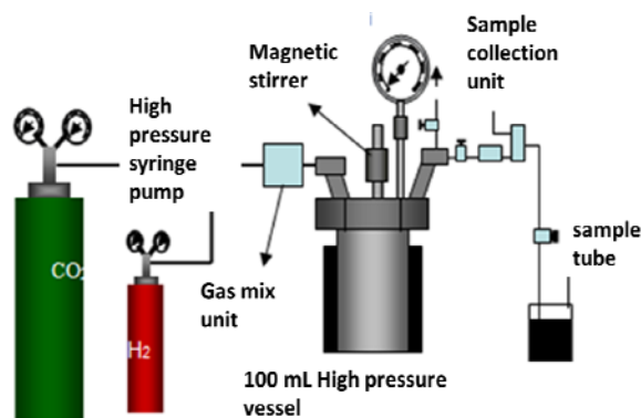
Fig. 4 SCF deposition apparatus
