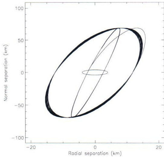
Fig. 15 (d) Scenario 4 – Change e_x and e_y and date of correction
