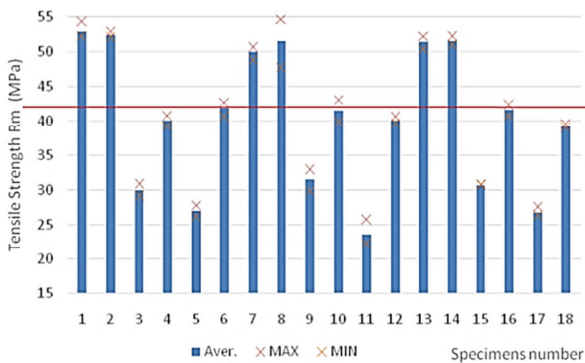
Fig. 9 Tensile Strength values
