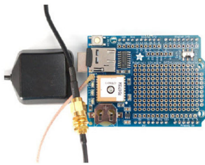
Fig. 7 Adafruit ultimate GPS data logger
