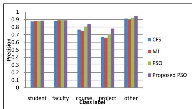
Fig. 3 Precision
