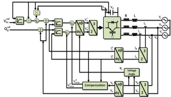
Fig. 14 Grid side VSR
