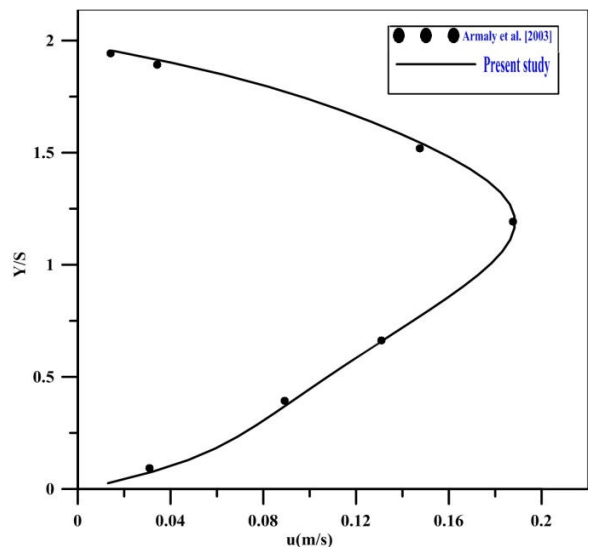
Fig. 2 (d) Profile of velocity at X/S=7
