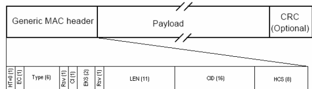
Fig. 2 IEEE 802.16 WMAN MAC PDU format
