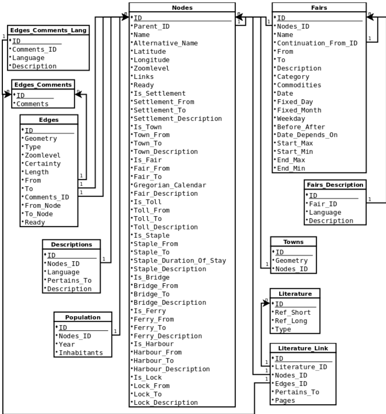
The Viabundus database schema.
