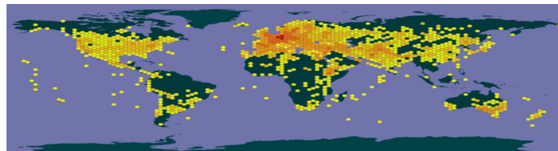
Рис. 5. Карта распространения представителей рода Triticum L. (GBIG)
