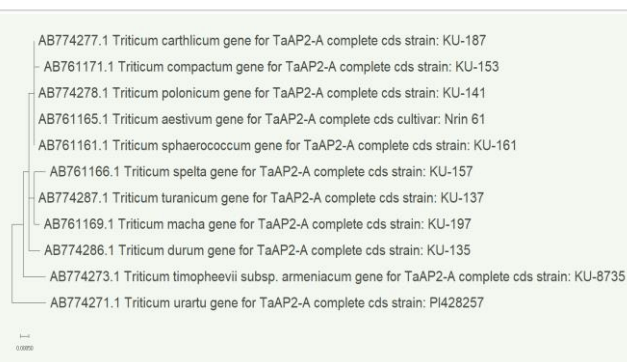
Рис. 3. Филогенетическое дерево рода Triticum L.
