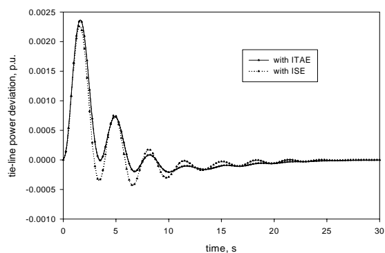
Fig. 6 (d) Tie-line power deviation in Area-3
