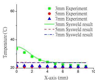
c) y=8mm
