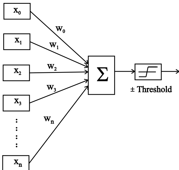
Fig. 2 Perceptron
