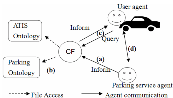
Fig. 3 Ontology update
