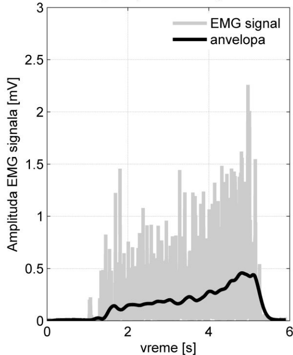
Dvostrano ispravljen EMG signal i anelopa
