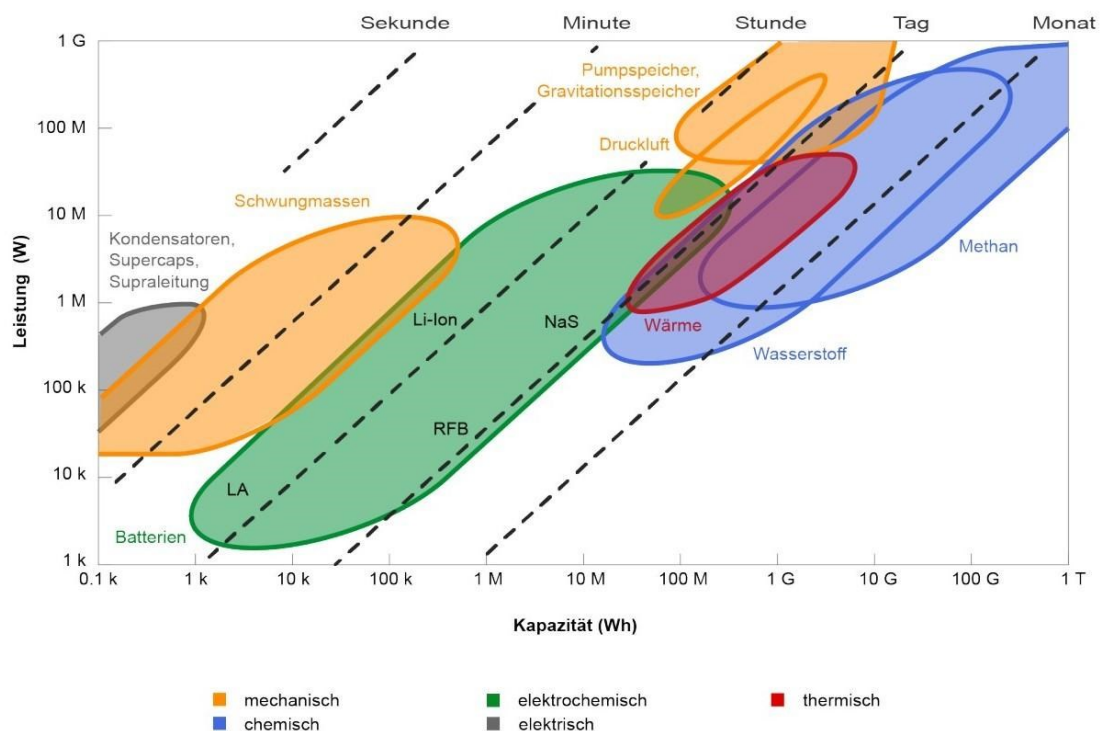
Abbildung 2: Schematische Übersicht zu Leistung und Energie (Kapazität) verschiedener Speichertypen (mechanisch, chemisch, elektrochemisch, elektrisch und thermisch). Mögliche Speicherzeiten liegen zwischen Sekunden und mehreren Monaten. Speziell gewisse Wärme- und Gasspeicher (Wasserstoff, Methan) sind interessant für saisonale Energiespeicherung über mehrere Monate. (Li-Ion: Lithium-Ionen-Batterien, NaS: Natrium-Schwefel-Batterien, LA: Bleibatterien (lead-acid battery), RFB: Flussbatterien (redox-flow battery). Quelle: (Oberholzer 2021).
