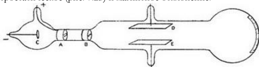
Рис. 7.23. Трубка Дж. Дж. Томсона для электростатического отклонения катодных лучей (J. J. Thomson 1897c). Отклоняющий потенциал приложен к пластинам D и E.
