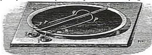
Рис. 1.13. Устройство для демонстрации взаимного отталкивания частей прямолинейного тока (Ампер 1822с). Токи в сегментах qr и pn плавающего провода отталкивают токи rs и nm в ртутной ванне
