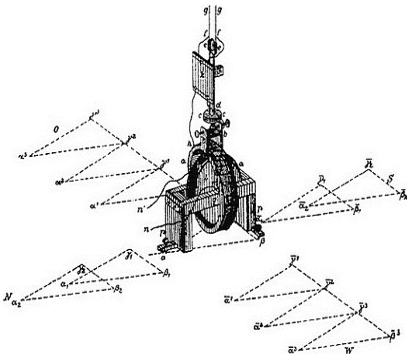
Рис. 2.4. Разделяемый электродинамометр (Weber 1846: 28). Бифилярная катушка А-А-А удерживается в постоянном положении. Статическая катушка III может перемещаться в разные положения a \beta \gamma
