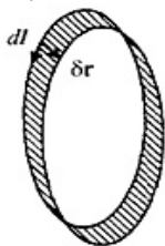
Рис. А.4. Деформация поверхности.
