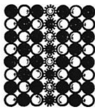
Рис. 5.7. Иллюстрация Лоджа прямого и обратного токов в двух проводниках, (круглые колеса), разделенных тонким изолирующим слоем. (зубчатые колеса) (Lodge 1889:189)
