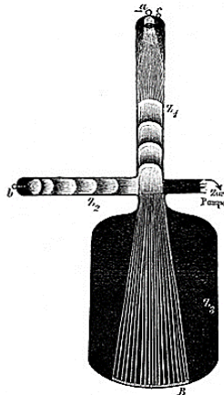
Рис. 7.10. Трубка Гольдштейна для демонстрации взаимной независимости различных слоев разряда (Goldstein 1880a). Лучи из пятого слоя направляются прямо во флуоресцентный экран B, даже, если анод находится в перпендикулярном направлении.
