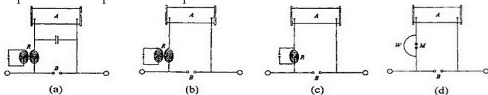
Рис. 6.10. (a), (b), (c), (d). A обозначает катушку Румкорфа, B - разрядник, R - спираль Рисса, M – микрометр Рисса
