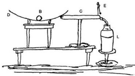
Рис. 3.5. Приспособление Фарадея, демонстрирующее индукцию при отсутствии заряженного тела (FD 2: 417).
