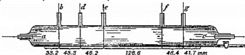
Рис. 7.8. Трубка Хиттона для измерения падения потенциала (Hitton 1883).
