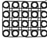
Рис.5.5. Моделирование Фицджеральдом электромагнитного поля резиновыми лентами (из Hunt 1991a: 79)
