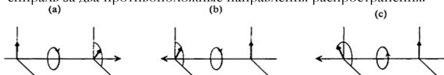
Рис. 3.24. Вращение плоскости поляризации света, проходящего через токовую петлю.
