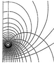
Рис. 4.2. Магнитные силовые линии и эквипотенциальные поверхности кругового тока, в полуплоскости, ограниченной осью круга (Максвелл 1873а: пластина 18).
