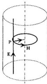
Рис. 5.2. Электрическая и магнитная силовые линии проходят через точку Р цилиндрического проводника. Стрелка в точке Р указывает направление потока энергии.
