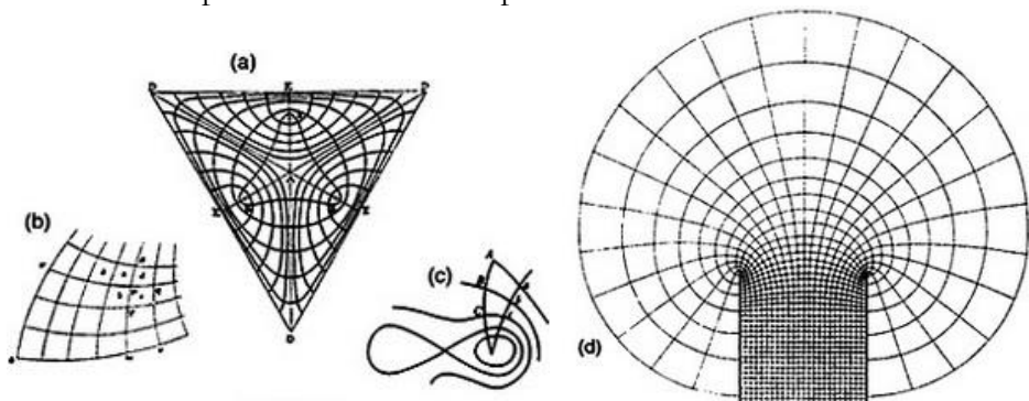
Рис. 4.1. Некоторые из геометрических сеток Максвелла:
