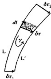
Рис. А.3. Деформация линии L .
