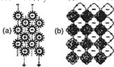
Рис. 5.6. Плоская модель эфира в виде зубчатых колес (а) и её улучшенная версия (b) (Lodge 1889: 179,180)
