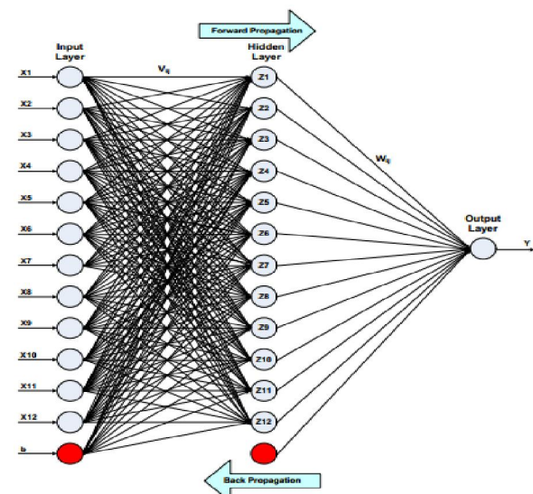
Gambar 2. Arsitektur Jaringan Saraf Tiruan Yang Digunakan
