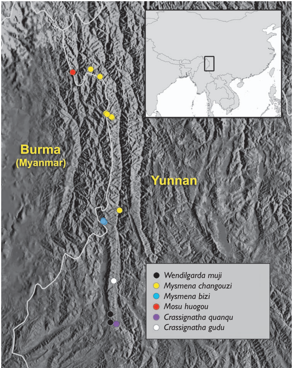
Figure 96. Distribution map, inset map shows study area. Black: Wendilgarda muji sp. n.; yellow: Mysmena changouzi sp. n.; blue: Mysmena bizi sp. n.; red: Mosu huogou sp. n.; purple: Crassignatha quanqu sp. n.; white: Crassignatha gudu sp. n.
