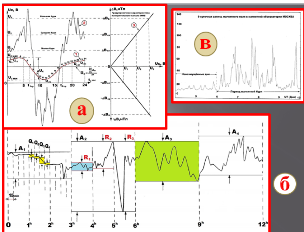
Рис.4. Пример установки измерителя ИМБ относительно ПММ (а), а также пример определения индексов магнитной активности (б) и фрагмент реальной записи Rh-индекса (в) при помощи ИМБ в период регистрации МБ на ЦМО МОСКВА.
