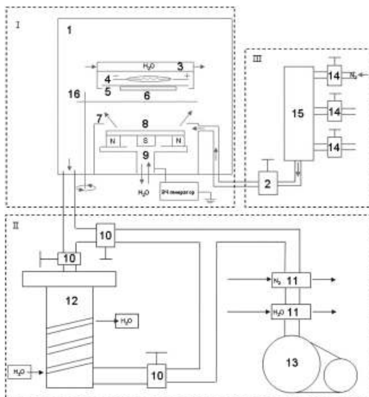
Рис. 1. Установка высокочастотного магнетронного напыления: 1 — рабочая камера; 2 — напускатель рабочего газа; 3 — охладитель подложкодержателя; 4 — нагреватель подложки; 5 — держатель подложки; 6 — подложка; 7 — анод; 8 — мишень; 9 — магнетрон; 10 — сильфонный клапан; 11 — азотная и водяная ловушки; 12 — диффузионный насос; 13 — форвакуумный насос; 14 — игольчатые клапаны натекания; 15 — смеситель газов; 16 — заслонка.
