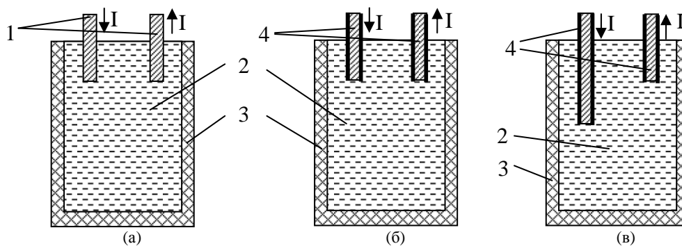
Рис. 1. Электродные системы для КЭТО: (а) с неизолированными равнозаглубленными электродами; (б) с изолированными равнозаглубленными электродами; (в) с изолированными разнозаглубленными электродами: I – неизолированные электроды; 2 – расплав; 3 – неэлектропроводная емкость с расплавом; 4 – электроды с изолированной боковой поверхностью.
