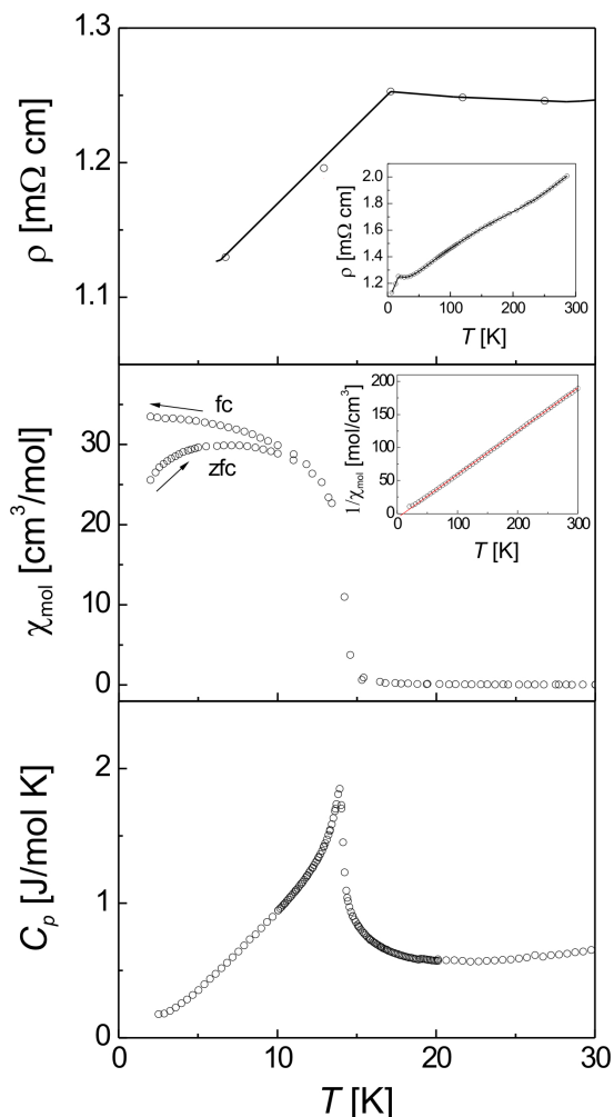
Abb. 2. Physikalische Eigenschaften von Pr 2 CBr. Oben: Temperaturabhängigkeit des elektrischen Widerstands \rho [m \Omega cm] im Bereich 6 \text{ K} \leq T \leq 30 \text{ K} ; Einschub 6 \text{ K} \leq T \leq 300 \text{ K} ; Mitte: Temperaturabhängigkeit der magnetischen Suszeptibilität \chi_{\text{mol}} [cm 3 mol -1 ] im Bereich 6 \text{ K} \leq T \leq 30 \text{ K} . Es sind die Abkühl- [mit äußerem Feld (fc)] und Aufheizkurven [ohne äußeres Feld (zfc)] gezeigt. Der Einschub zeigt die reziproke Molsuszeptibilität 1/\chi_{\text{mol}} [mol cm -3 ] im Bereich 6 \text{ K} \leq T \leq 300 \text{ K} ; unten: Temperaturabhängigkeit der spezifischen Wärme C_p [J mol -1 K -1 ] im Bereich 6 \text{ K} \leq T \leq 30 \text{ K} .
